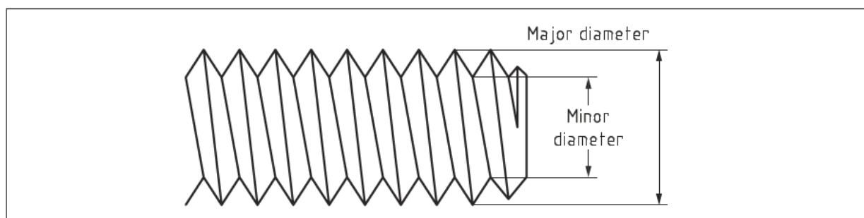
شکل ج-۱- جزئیات رزوه معمولی که قطرهای بزرگ و کوچک را تعریف می‌کند.
