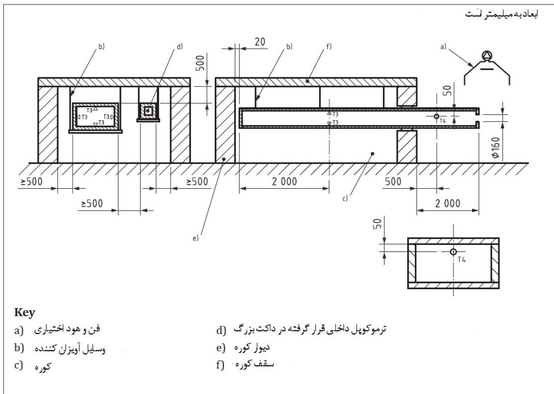
شکل چ-۱- نمونه آرایش آزمون برای داکت‌های عمودی (در معرض آتش خارجی)،
