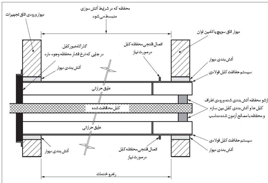
شکل ۳- جزئیات دیوار- محفظه کابل
