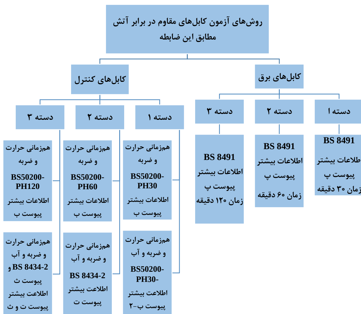
شکل ۲- روش‌های آزمون کابل‌های مقاوم در برابر آتش (کابل‌های برق- کابل‌های کنترل)
