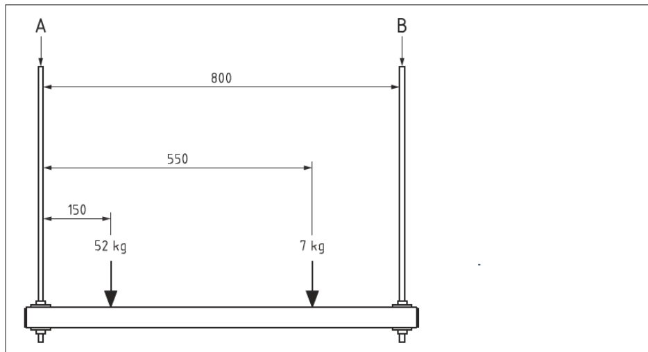
شکل ج-۳- مثال بار مکانیکی بر آویز نگهدارنده
